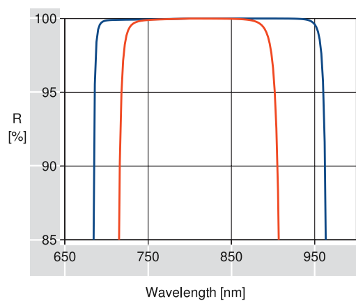
BROADBAND H.R. COATING R59: 770-830nm S-POL, 45° ——— P-POL, 45° ———
