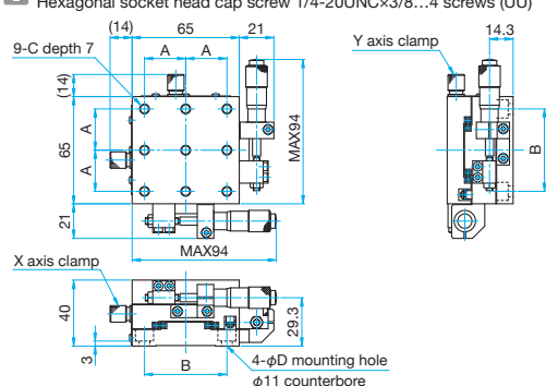
TAM-652S-M6/652SUU
